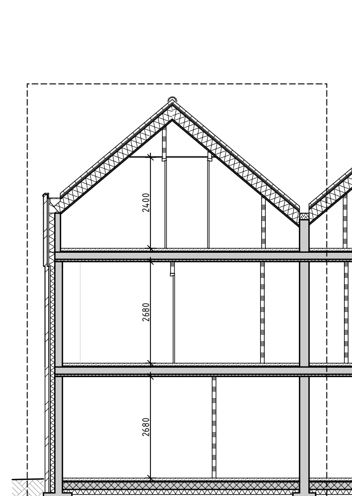
doorsnede A-A
