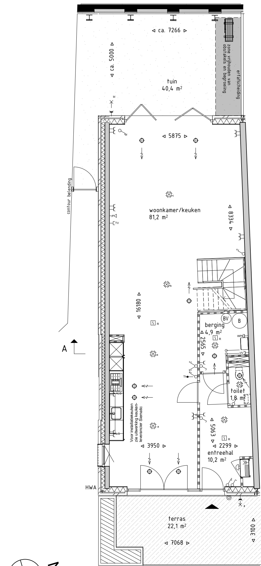
begane grond
